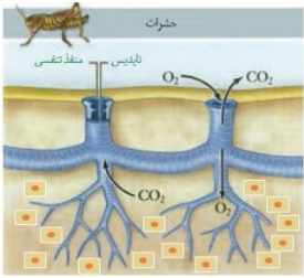
شکل ۲۱- تنفس نایدیسی
