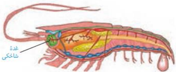
شکل ۱۵- غدد شاخکی
