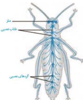
پ) ملخ
